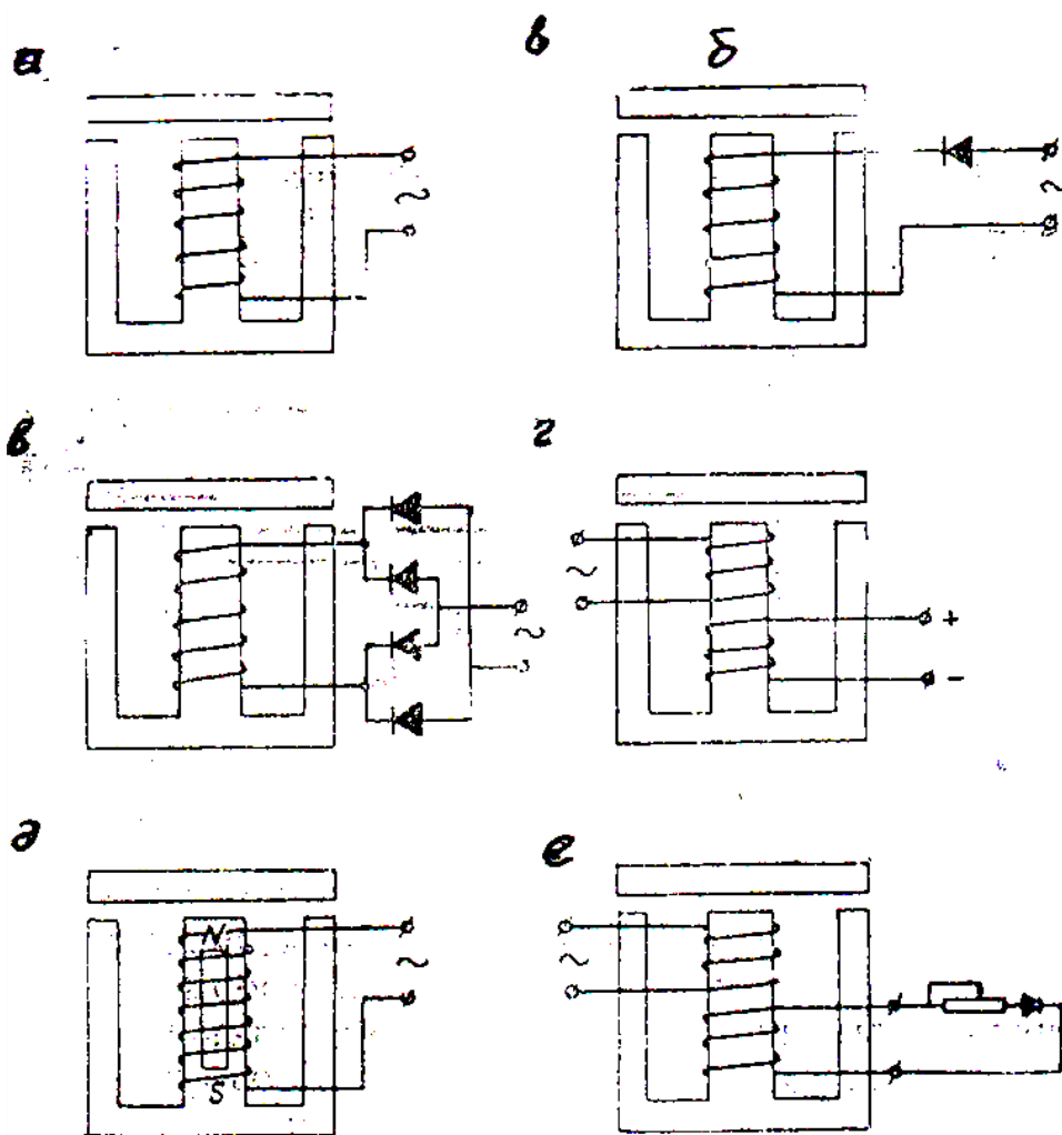
Рис.1. Схемы однотактных вибрационных возбудителей
