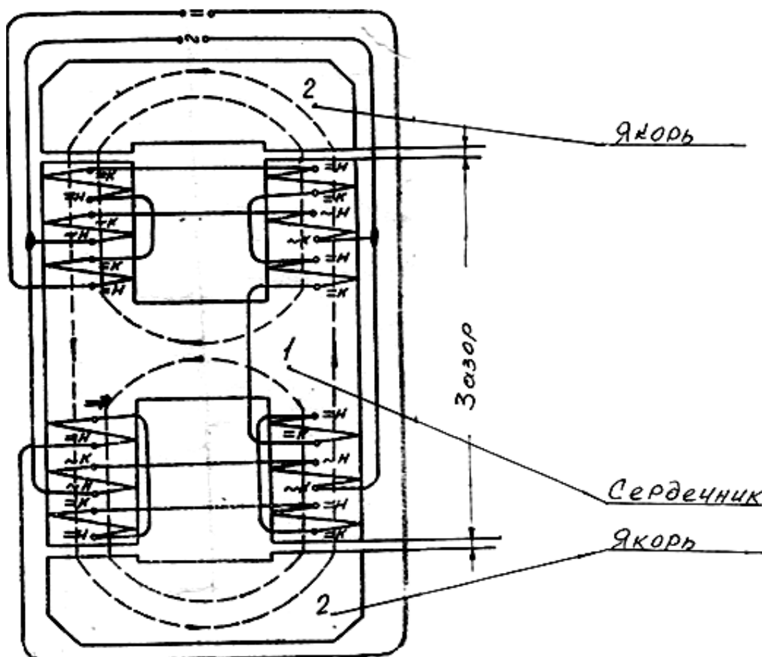
Рис. 2. Схема электромагнита с поперечным зазором между сердечником и якорями
