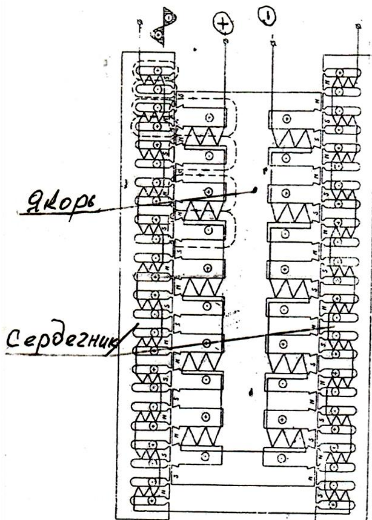
Рис. 3. Схема электромагнита электровибрационного двигателя с продольным зазором магнитопровода
